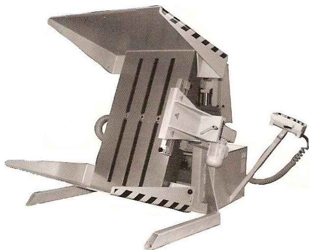
РТ10 РАЈ с раздухващо и вибриращо устройство
